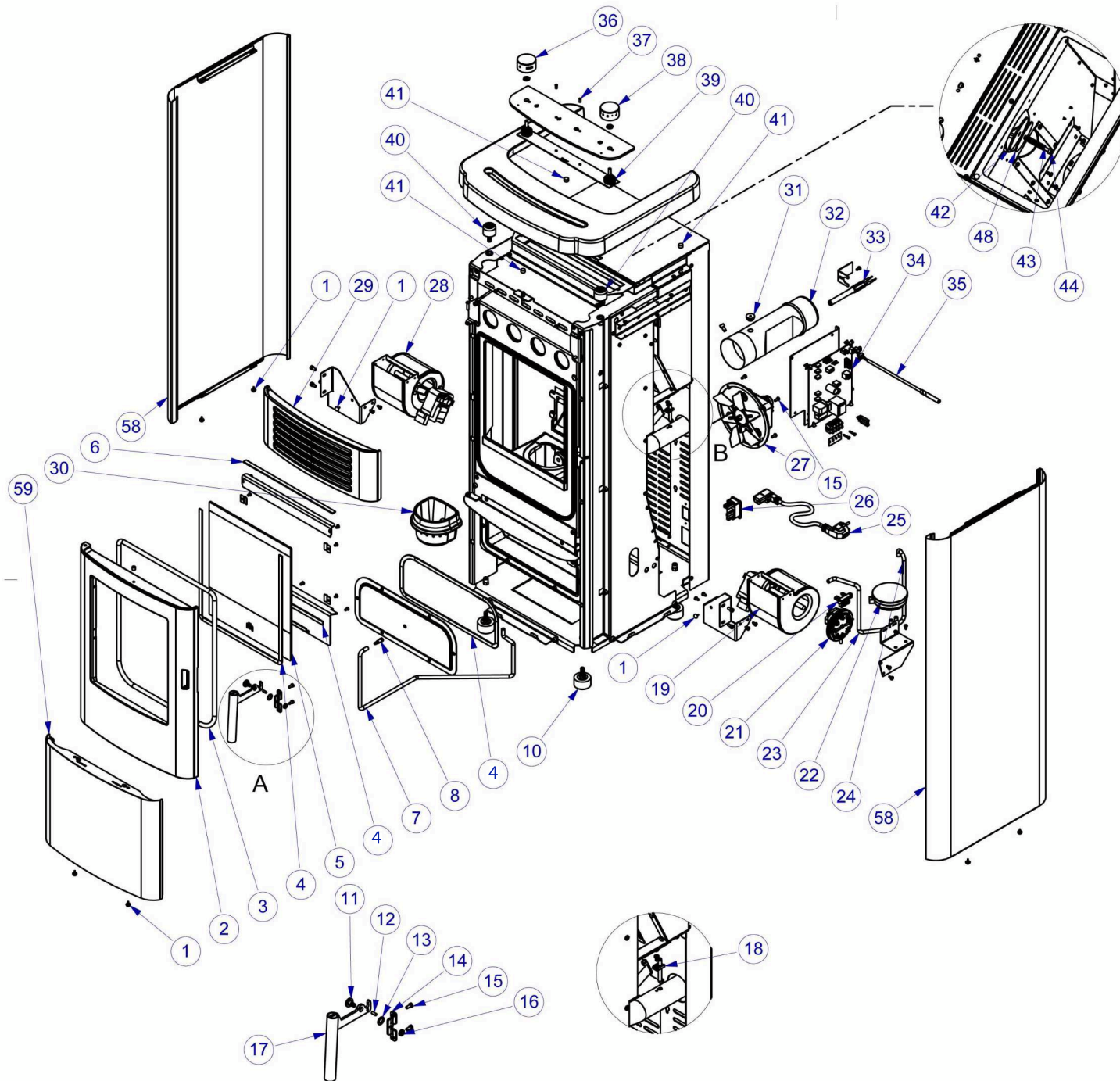
DETTAGLIO A SCALA 2 : 15
