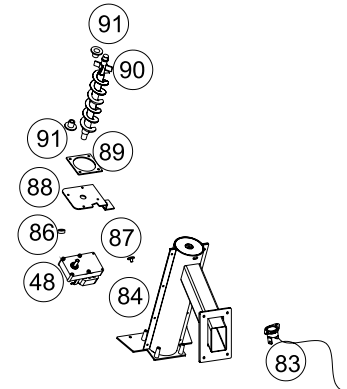
Assieme caricatore cod.249960
